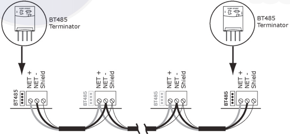
Fig. 24 — Network Wiring
