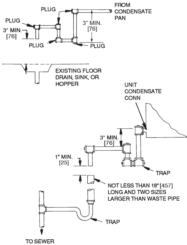
Fig. 12 - Condensate Drains
