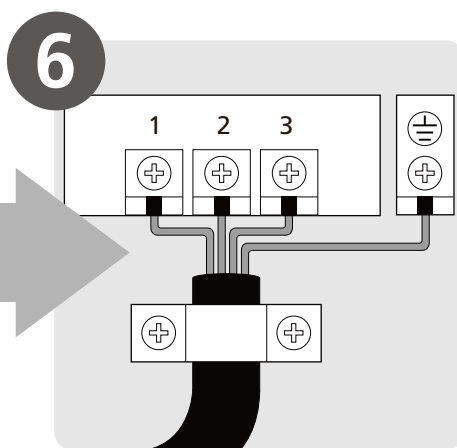
6 Conecte el cableado (Página 17)
