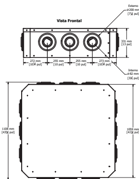
Pleno difusor de aire por los 4 lados
