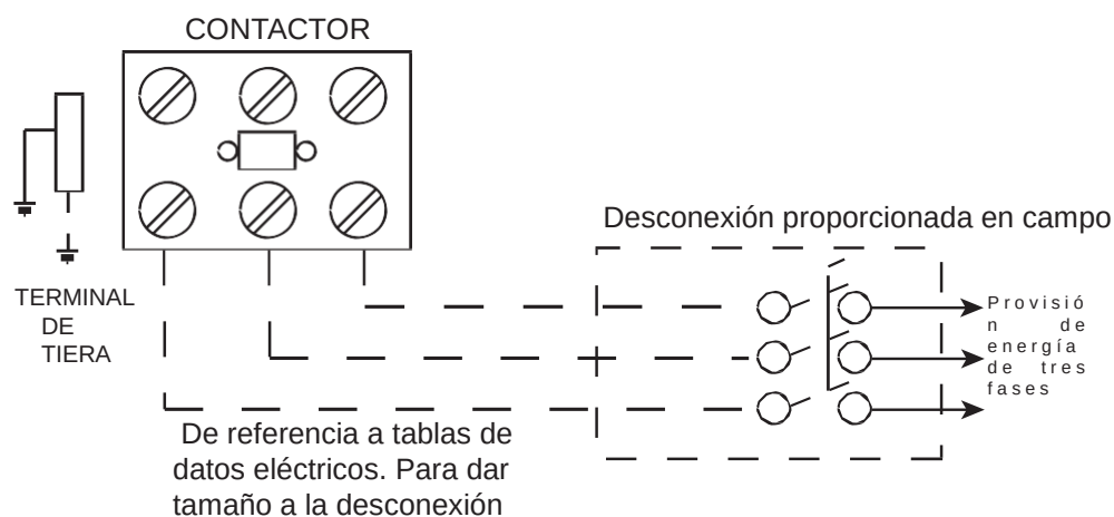
Fig. 6-2 Diagrama de Cableado de Energía de Campo Típico (Continuación)
