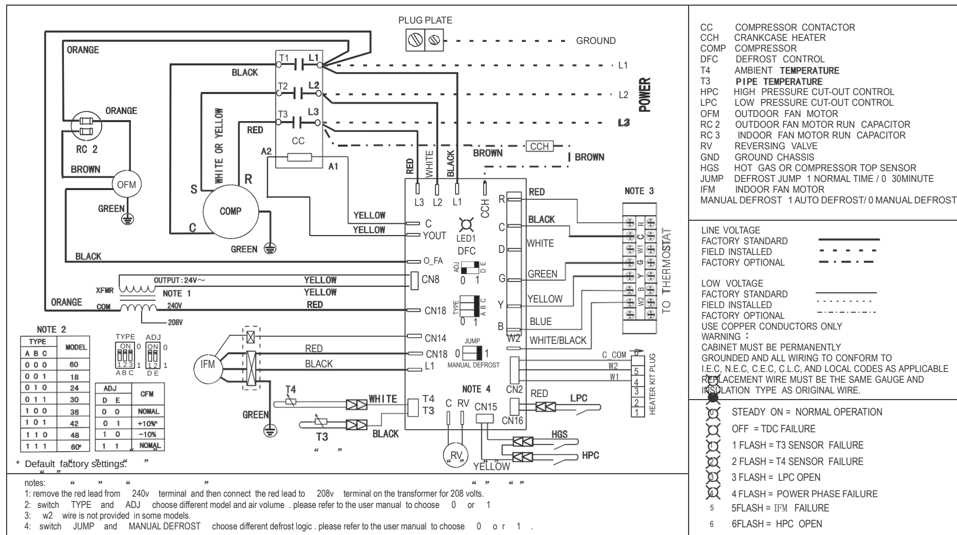
Diagrama de Cableado de Sistema HP (60K 3 fase)
