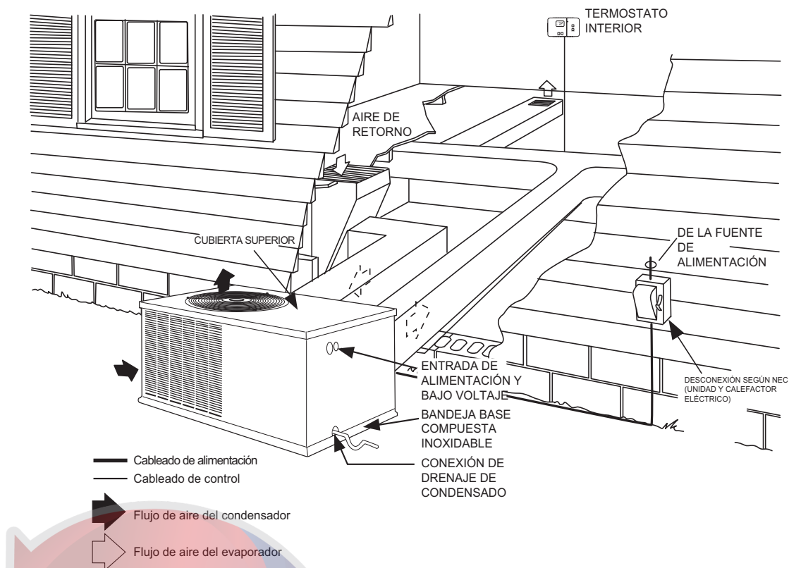
Fig. 7 – Instalación típica
