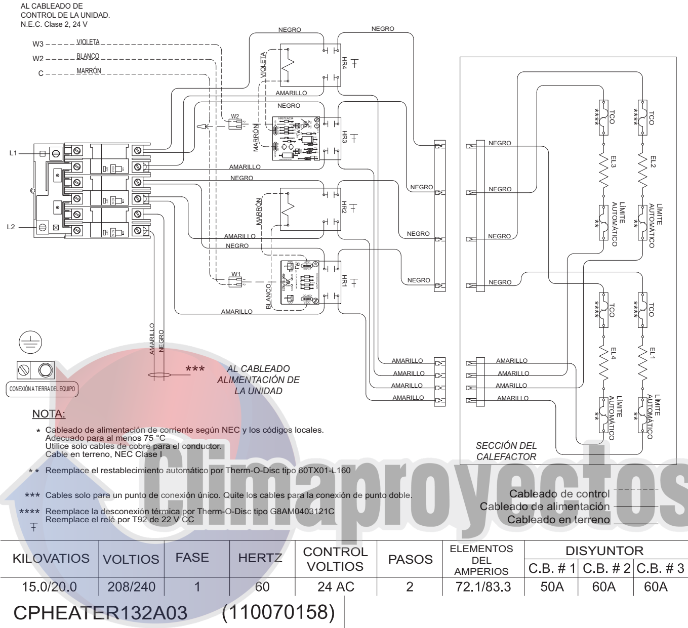
Fig. 16 – Cableado de calefacción eléctrica auxiliar monofásico
